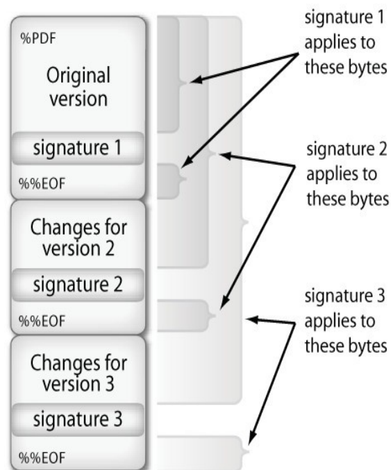
Figura 8: Assinatura Incremental em PDF
