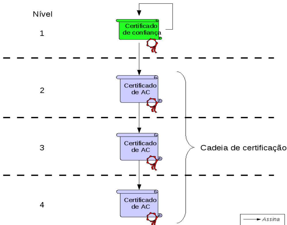
Figura 1: Exemplo de uma cadeia de certificação da ICP-Brasil
